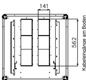
Ansicht Schrankboden
