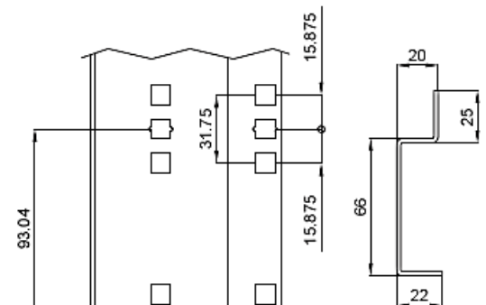
19" Profilschienen
